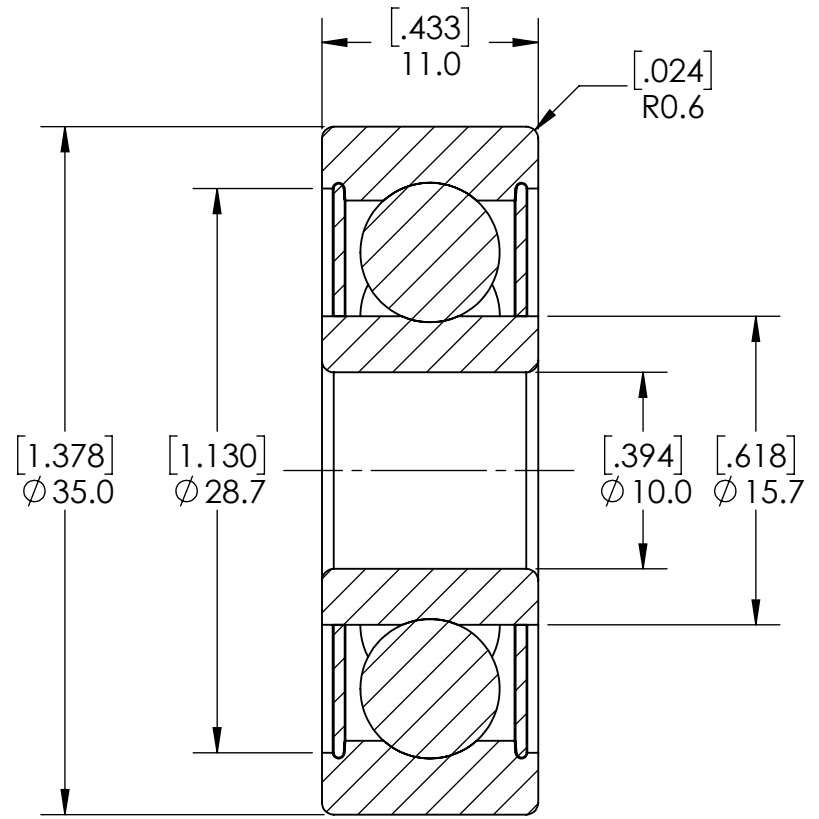
SECTION A-A
